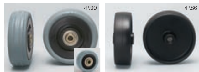
(LDA/LMDA用) VPA Kゴム(SBR) ●ベアリング入 (LDA/LMDA用) POA Gナイロン(ナイロン6) ●カラー入
