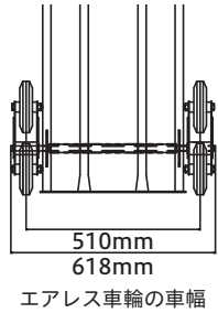
エアレス車輪の車幅
