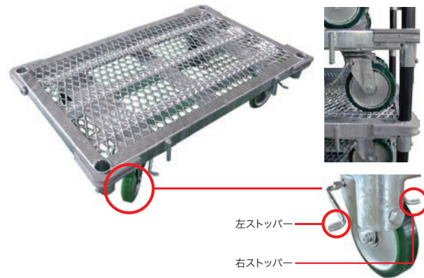
スタンダードプレスキャストストッパー付 (ウレタン車輪)
